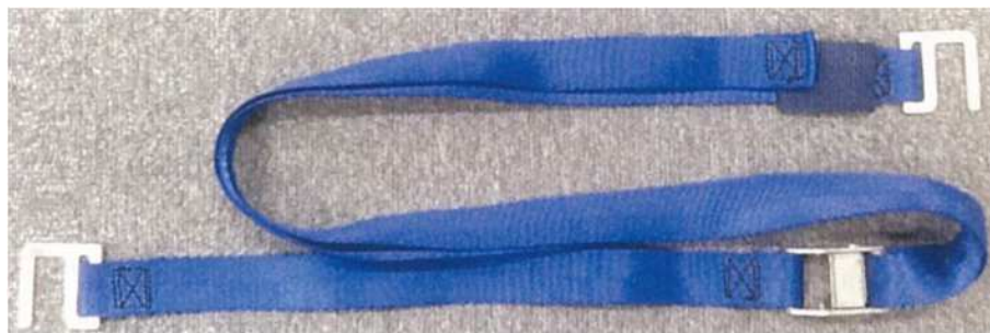
カム式ドロップフック 破断強度 約250kg
