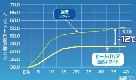
遮熱性能比較 (メーカー試験)
